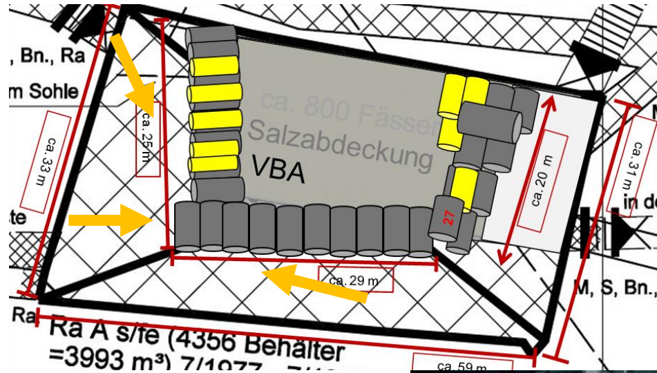
Schematische Einlagerung
